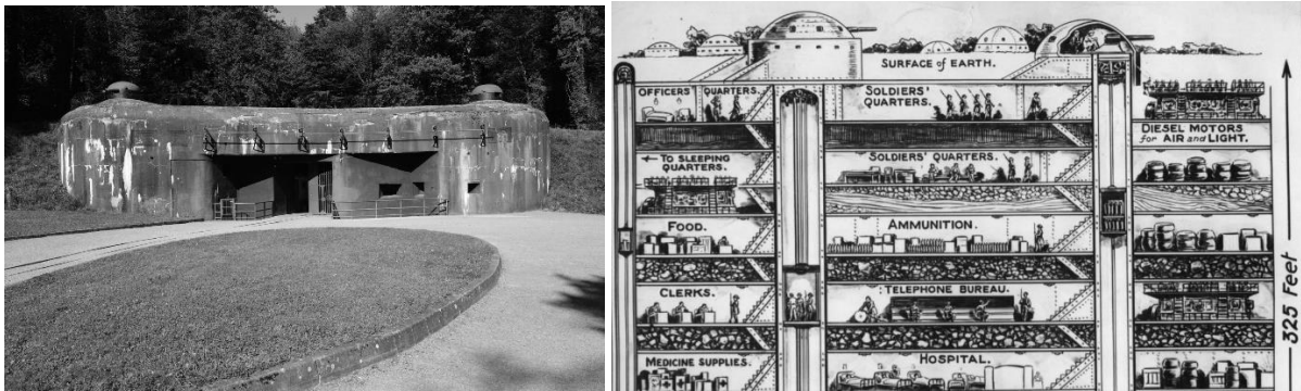
Vasbeton-erőd a Maginot-vonalban – Az erődök földalatti részének metszete
