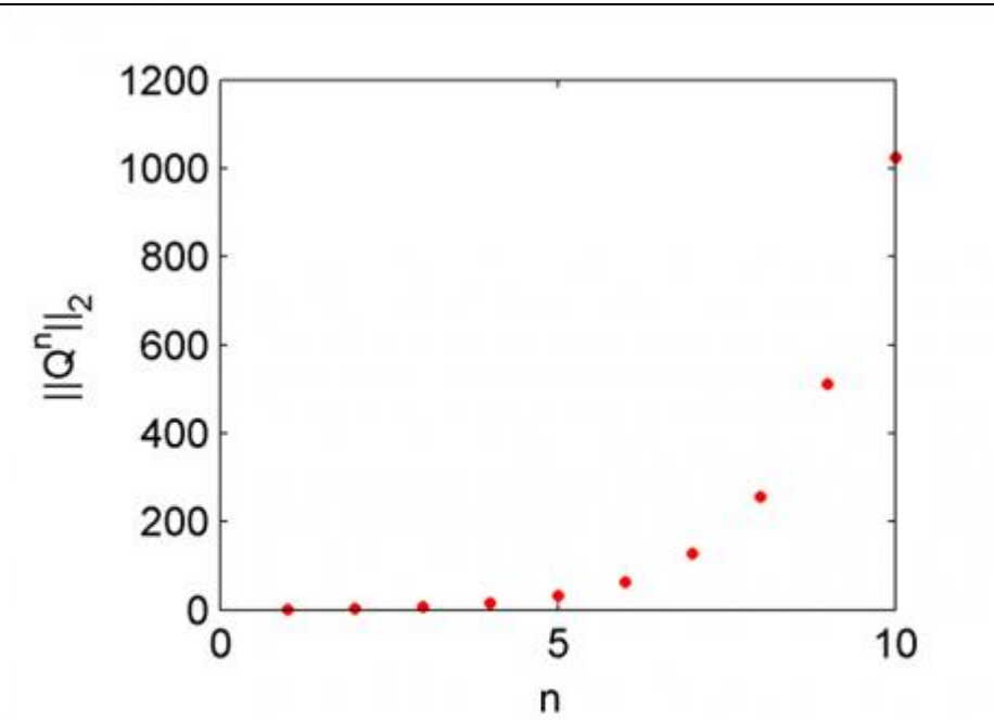
48. ábra. A \|Q^n\|_2 normák értéke n függvényében, ha r = \delta/h^2 = 1 (instabil eset), n\delta = 1 . Q az explicit Euler-módszer lépésmátrixa.
