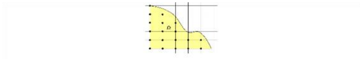
35. ábra. Egy lehetséges \Omega tartomány, a hozzá tartozó rácsháló és az \Omega_{\mathbf{h}} rácspontok halmaza.
