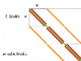
5. ábra. Az A_h mátrix szerkezete. Zöld: 2/h_1^2 + 2/h_2^2 , piros: -1/h_1^2 , narancs: -1/h_2^2 .
