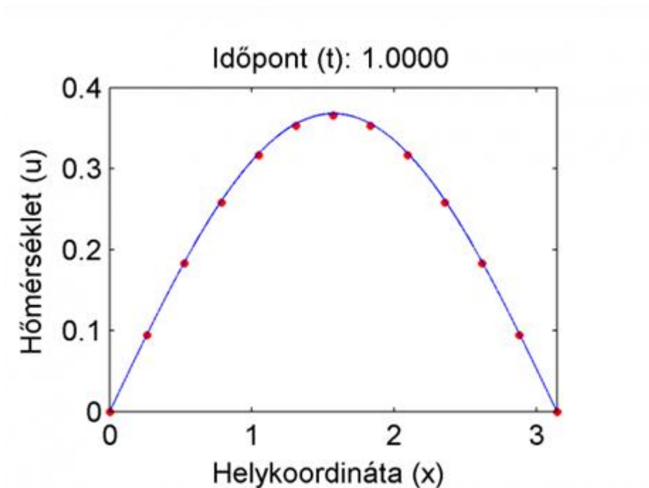
40. ábra. A (??) séma eredménye a t = 1 pontban (piros pontok). \sigma_D = 1 , h = \pi/12 , \delta = 0.025 . A pontos megoldást kék vonal szemlélteti. A legnagyobb eltérés értéke a középső rácspontban van, értéke 0.002518.
