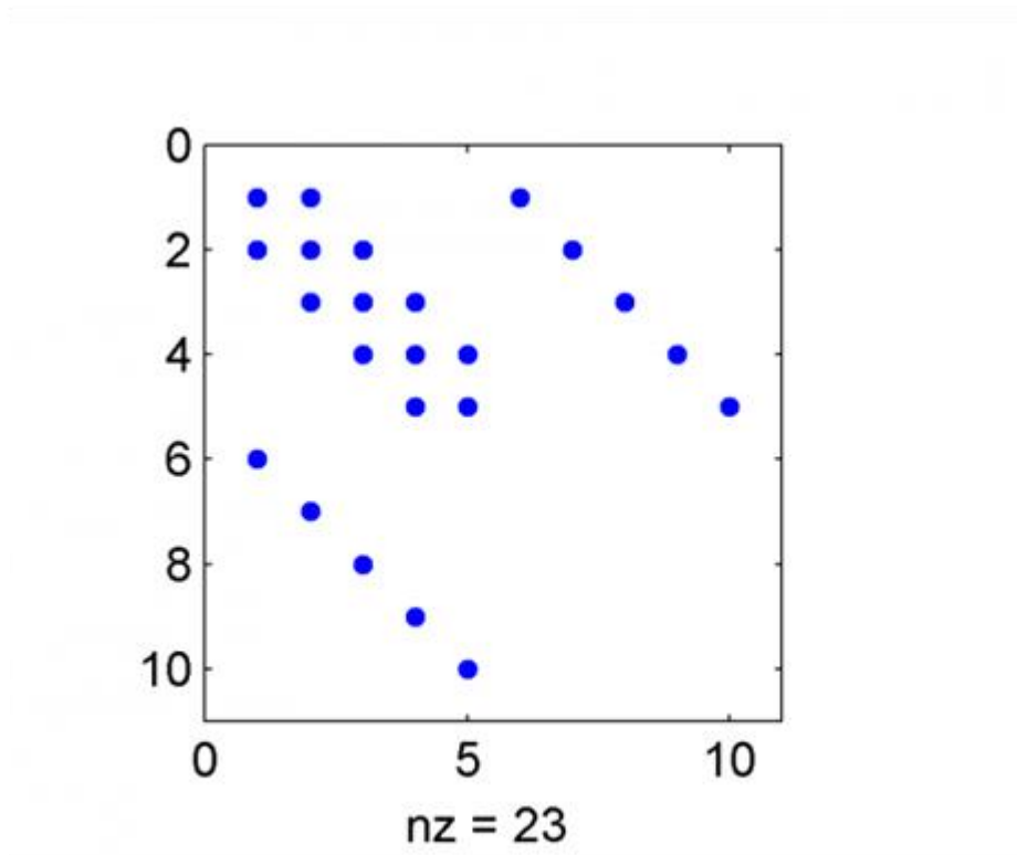
66. ábra. Nemnulla elemek a (??) sémához tartozó lépésmátrixban, ha a (??) feladatban nulla peremfeltételek adottak és az intervallumot hat egyforma hosszú részre osztottuk.
