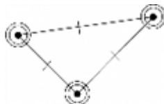
24. ábra. Argyris-elem.
