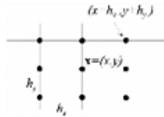
37. ábra. Az \mathbf{x} ponthoz és a D_{0,x}^2 D_{0,y}^2 véges differenciához tartozó alappontok.
