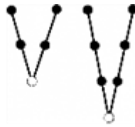
31. ábra. A V -ciklus szemléltetése három és négy rác esetén.
