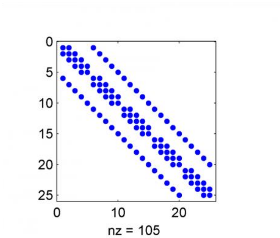
51. ábra. A nemnulla elemek elhelyezkedése a lépésmátrixban n_x = n_y = 5 esetén.
