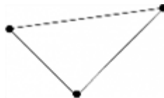
12. ábra. T_3 -elem (Courant-elem).
