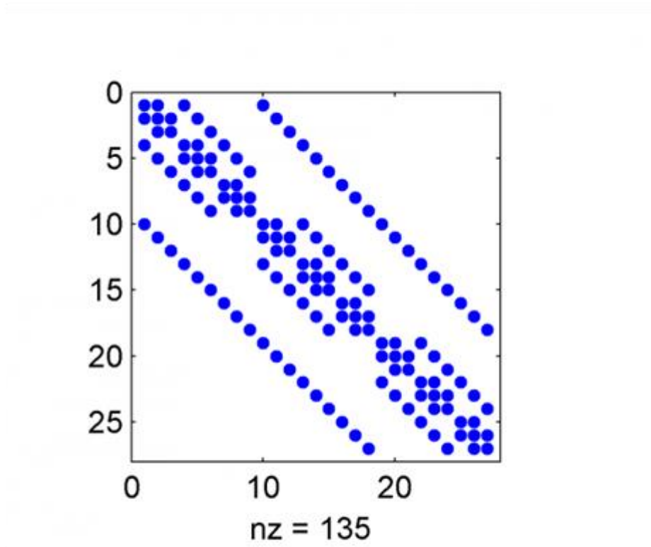
54. ábra. A háromdimenziós feladat Crank–Nicolson-sémájának bal oldalán álló I - \frac{r_x}{2} D_{0,x}^2 - \frac{r_y}{2} D_{0,y}^2 - \frac{r_z}{2} D_{0,z}^2 mátrix nemnulla elemek elhelyezkedése ( n_x = n_y = n_z = 3 ).
