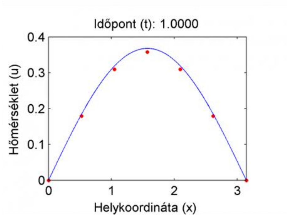
39. ábra. A (??) séma eredménye a t = 1 pontban (piros pontok). \sigma_D = 1 , h = \pi/6 , \delta = 0.1 . A pontos megoldást kék vonal szemlélteti. A legnagyobb eltérés a középső rácspontban van, értéke 0.01033.
