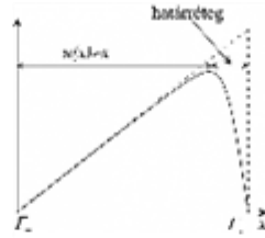
29. ábra. Konvekció-dominált 1D feladat megoldása.
