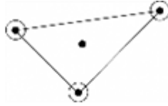
23. ábra. Kétdimenziós köbös Hermite-elem.
