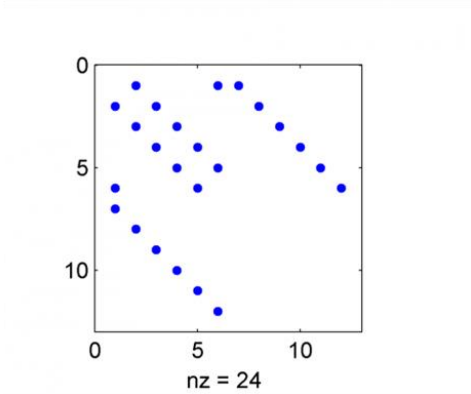
64. ábra. Nemnulla elemek a (??) sémához tartozó lépésmátrixban, ha a feladathoz periodikus peremfeltételek tartoznak és az intervallumot hat egyforma hosszú részre osztottuk.
