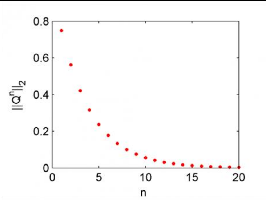
50. ábra. A \|Q^n\|_2 normák értéke n függvényében, ha r = \delta/h^2 = 1/4 (stabil eset), n\delta = 1 . Q az explicit Euler-módszer lépésmátrixa.
