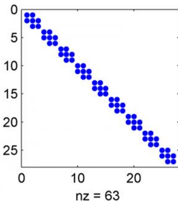
55. ábra. A háromdimenziós feladat Douglas–Gunn-sémájának bal oldalán álló I - \frac{r_x}{2} D_{0,x}^2 mátrix nemnulla elemeinek elhelyezkedése ( n_x = n_y = n_z = 3 ).
