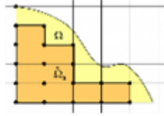
36. ábra. Az \tilde{\Omega}_h halmaz szemléltetése.
