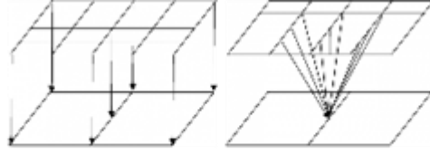
30. ábra. Restrikció téglalapprácson.
