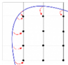
7. ábra. Peremértékek átvitele a rácspontokba.
