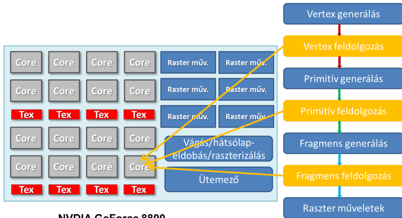
NVIDIA GeForce 8800 egységes shader GPU
