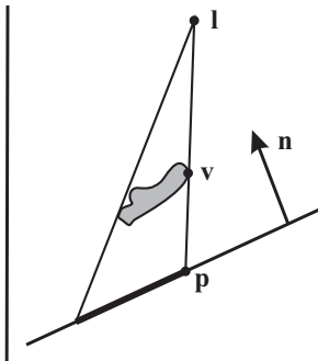
\pi : \mathbf{n} \cdot \mathbf{x} + d = 0 síkra vetett árnyék.
