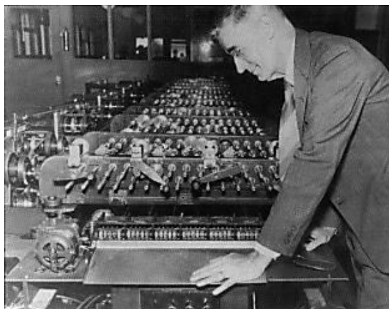
1.12. ábra. Univerzális analóg számítógép, MIT, 1930.
