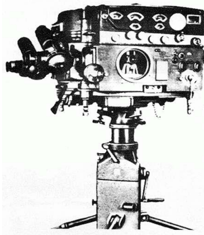
1.11. ábra. A Gamma-Juhász féle löelemképző készülék.
