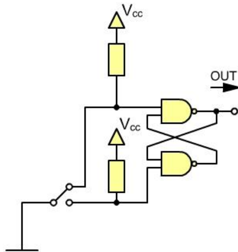
9.12. ábra. Információ olvasása érintkezőről, hardver pergesmentesítés.
