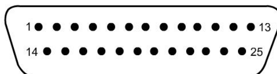
6.12. ábra. D25-ös RS-232C csatlakozó lábkiosztása.
