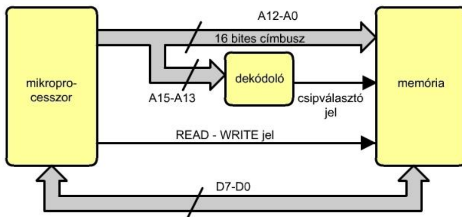
5.20. ábra: Példa a memória-választó logikára és címzésre, 8 kB memória esetén.
