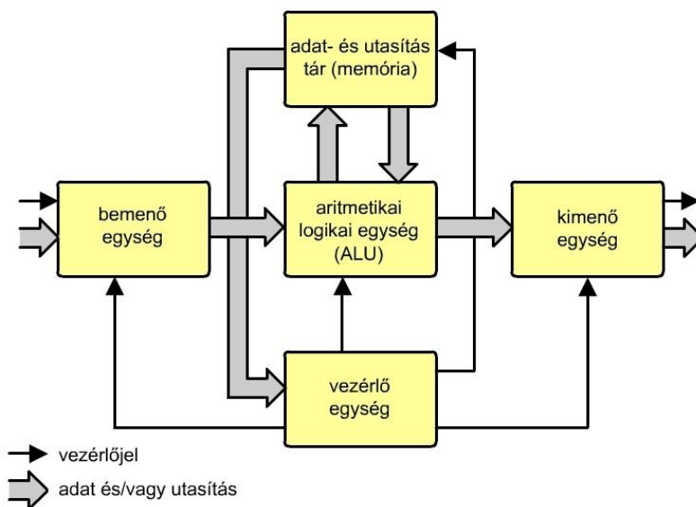
3.15. ábra. Neumann-féle számítógépmoell.
