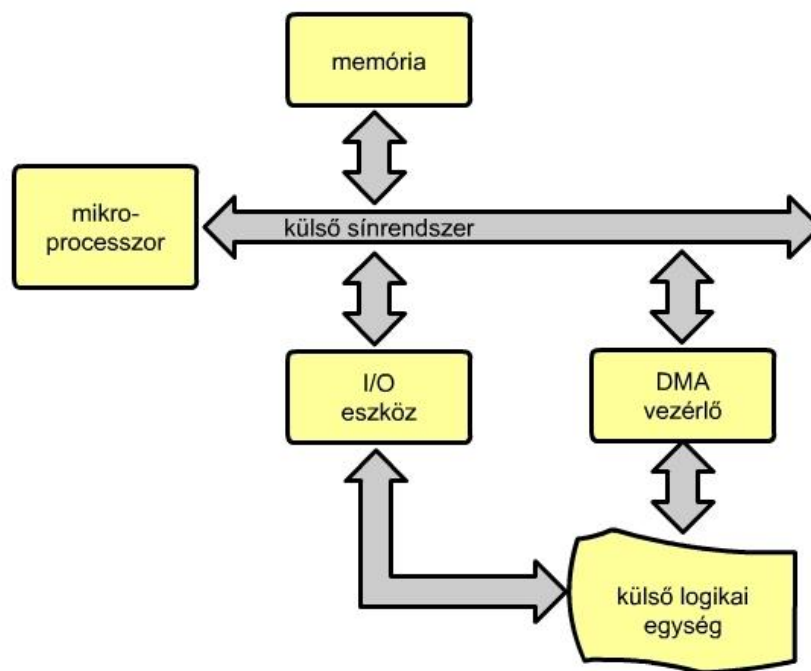
6.26. ábra. Egy valós, a meglevő sínrendszerre épülő DMA.
