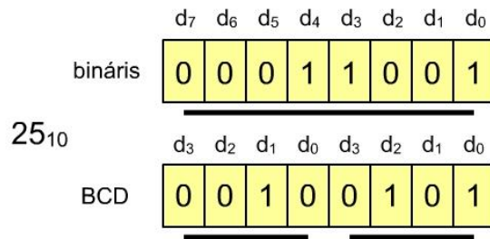
2.2. ábra. Példa egy tízes számrendszerbeli szám bináris és BCD ábrázolására.
