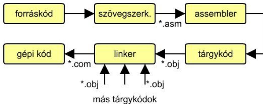
4.1. ábra. A prograrmírás, fordítás és szerkesztés folyamata.
