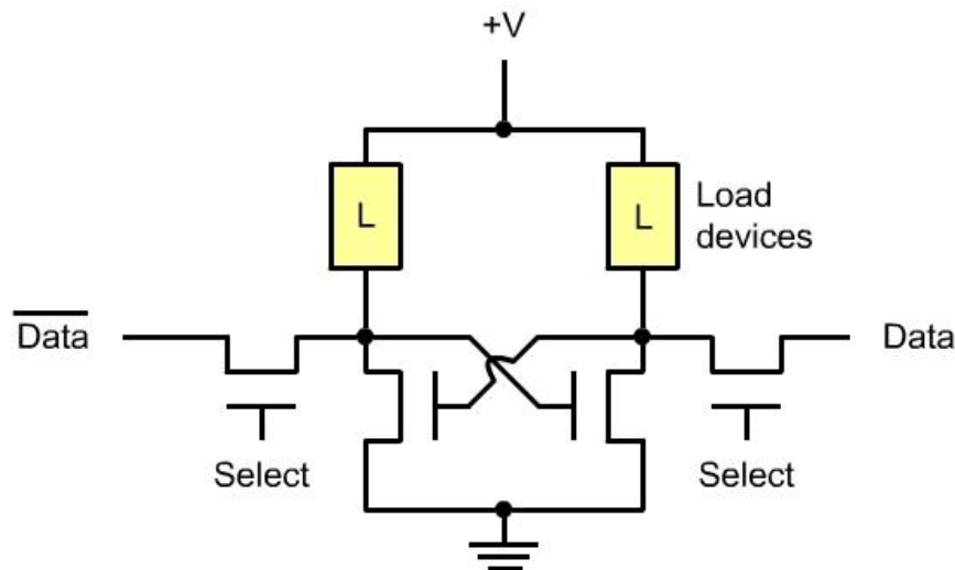
5.3. ábra. Statikus RAM kapcsolási rajza 4 tranzisztorral, 2 ellenállással.
