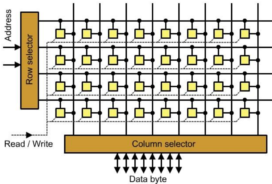
5.5. ábra. Statikus RAM szervezése.
