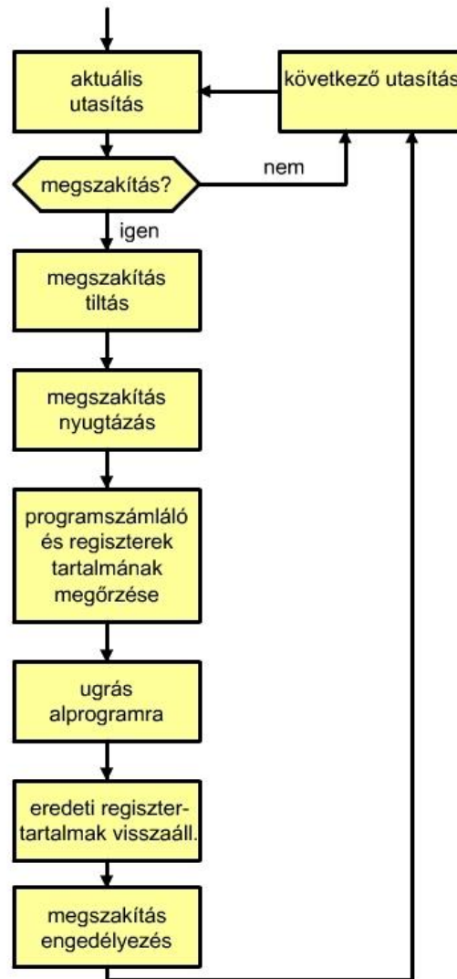
6.21. ábra. Megszakítással kezdeményezett adatátvitel folyamatábrája.
