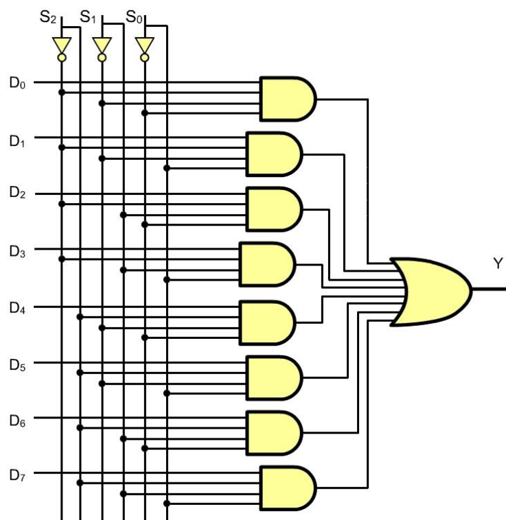
2.27. ábra. 8 bemenetű multiplexer felépítése logikai kapukkal.
