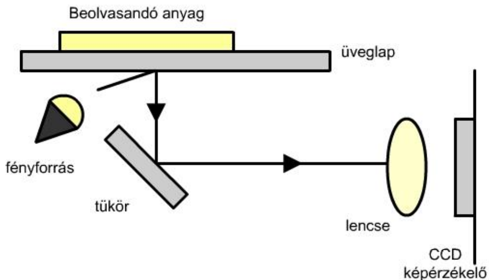
9.18. ábra. Síkágyas (asztali szkennер).
