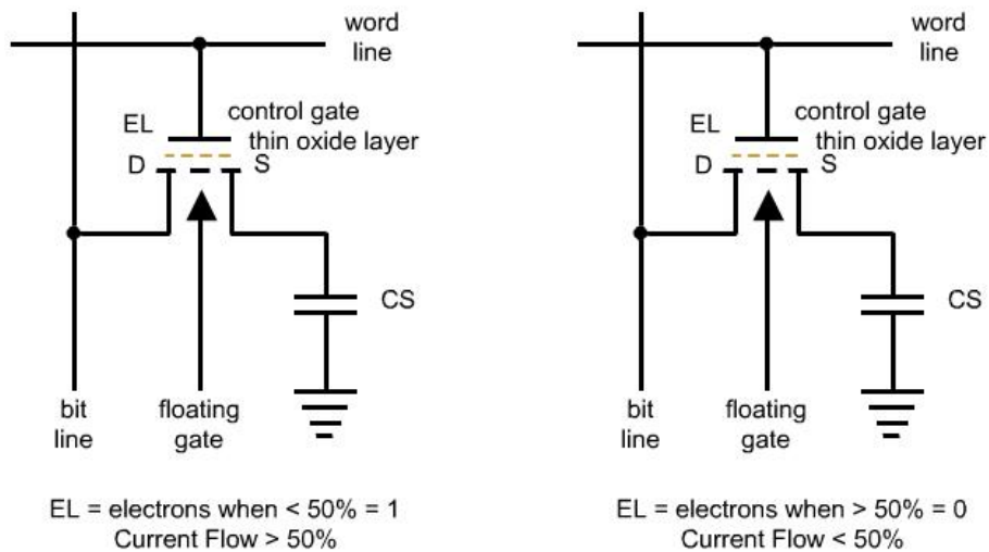
5.11. ábra. Írható-törölhető ROM, EPROM memória működése.
