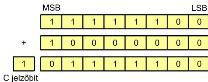
4.28. ábra. Példa olyan összeadásra, ahol átvitel keletkezik.
