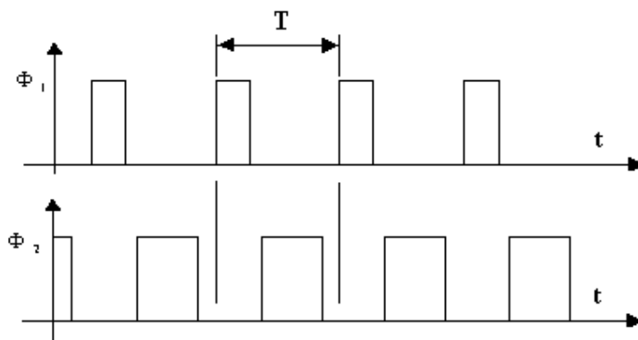
4.8. ábra. Kétfázisú órajel.
