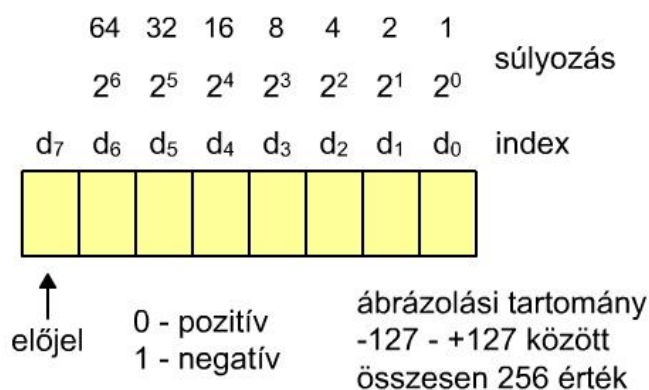
2.4. ábra. Pozitív és negatív egész számok ábrázolása.
