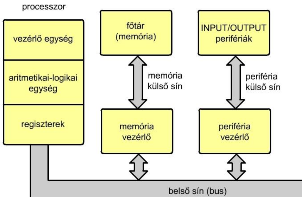
3.8. ábra. Memória- és perifériavezérlővel ellátott architektúra (külső sín).
