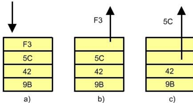
5.29. ábra: Példa a PUSH (a ábra) és a POP (b és c ábra) használatára
