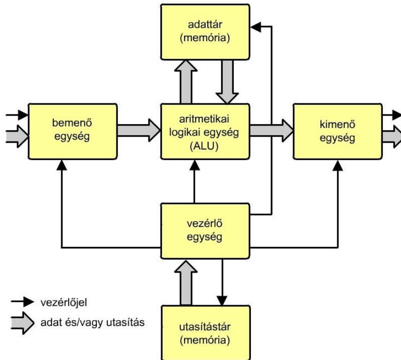
3.16. ábra. Harvard-féle számítógépmódel.
