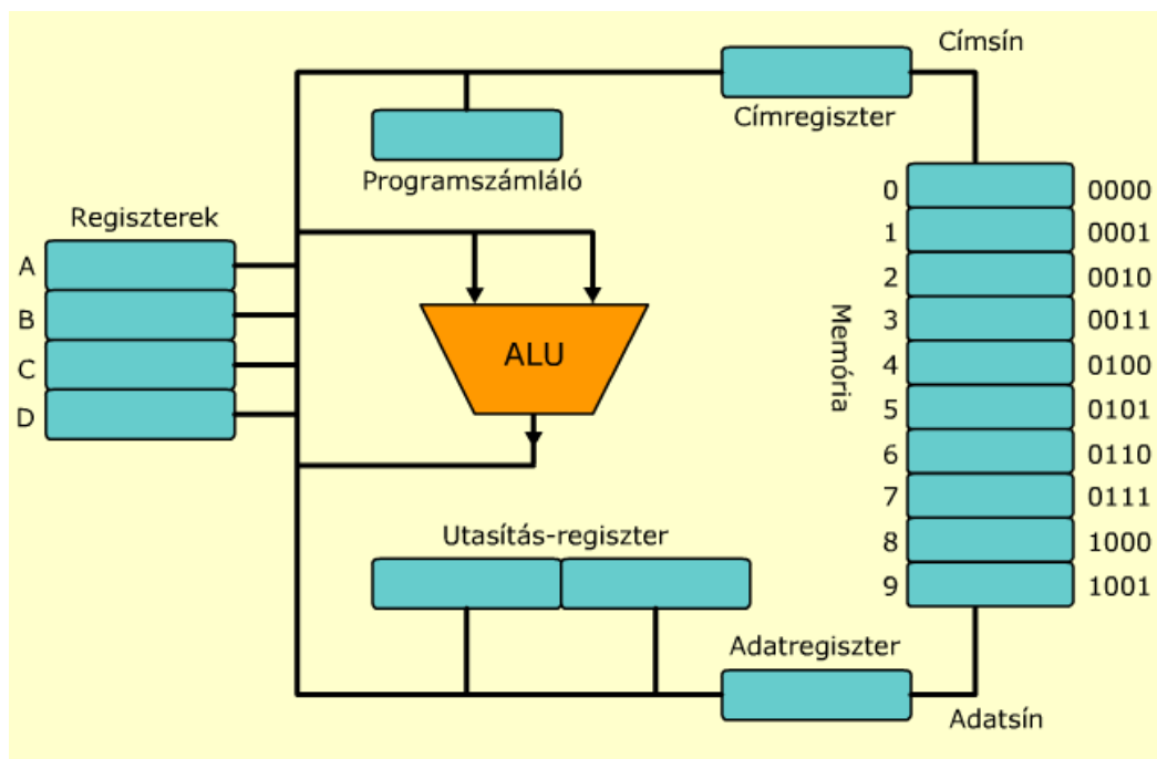
04.2. ábra. A számítógép-modell
