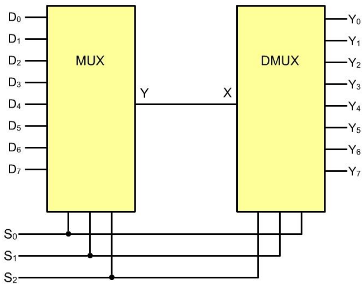
2.31. ábra. Multiplexer és demultiplexer összekapcsolása.
