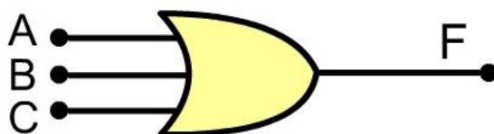
2.13. ábra. 3 bemenetű logikai VAGY kapu.
