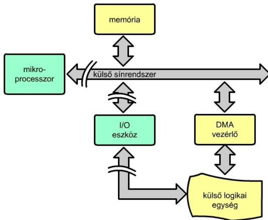
6.27. ábra. DMA adatátvitel.
