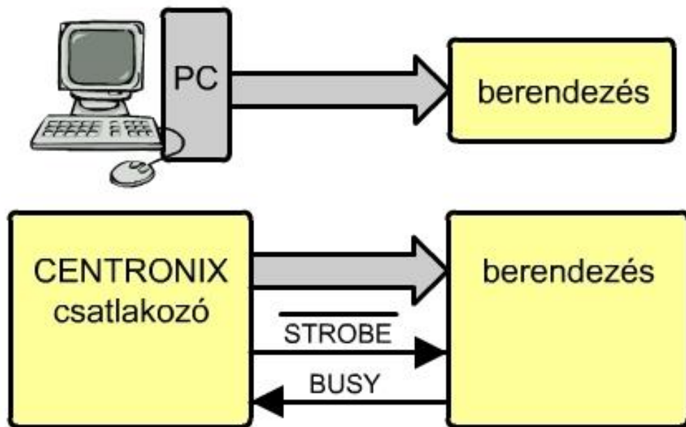
6.4. ábra. Párhuzamos adatátvitel PC-ből berendezésbe CENTRONICS párhuzamos csatlakozóval.
