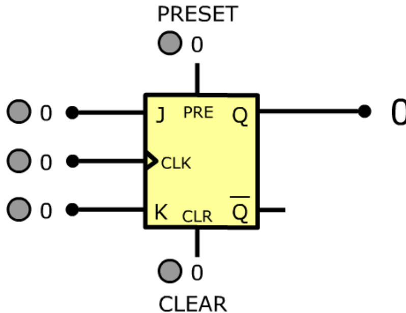
02.2. ábra. A JK tároló.
