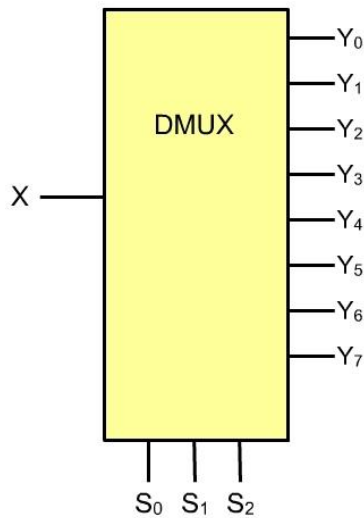
2.30. ábra. Demultiplexer szimbolikus rajzjele.
