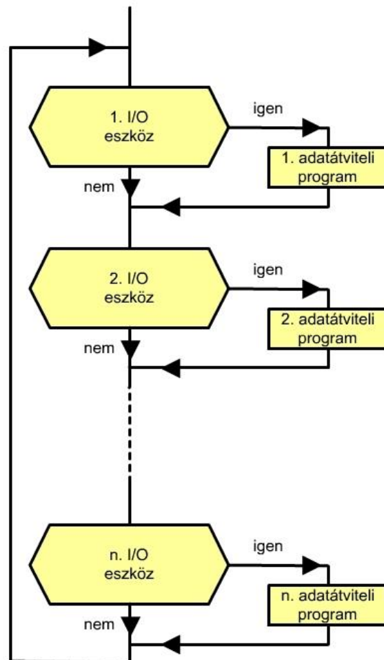
6.20. ábra. A kiválasztásos, feltételes ciklikus adatátvitel folyamatábrája.
