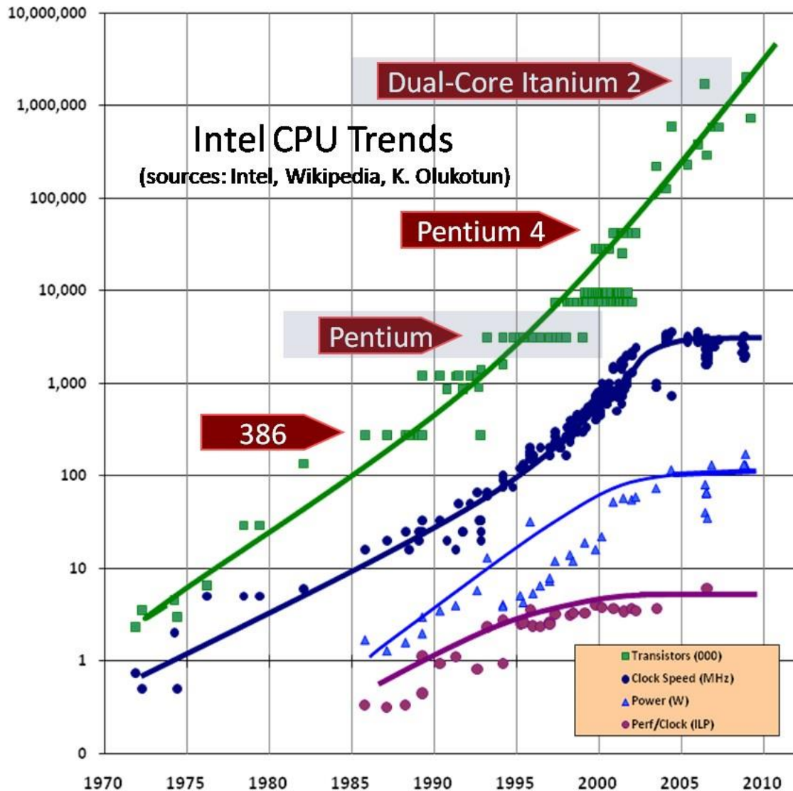
1.34. ábra. Moore törvénye órajellel és fogyasztással kiegészítve.
