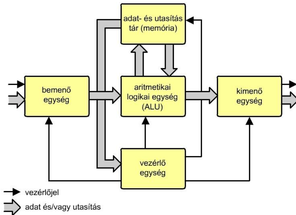
3.9. ábra. Egyszerű Neumann modell.
