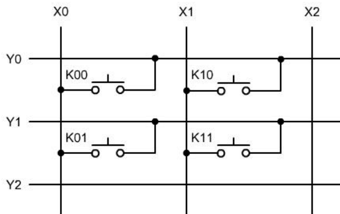
9.15. ábra. Klaviatúra-mátrix kapcsolási rajza.
