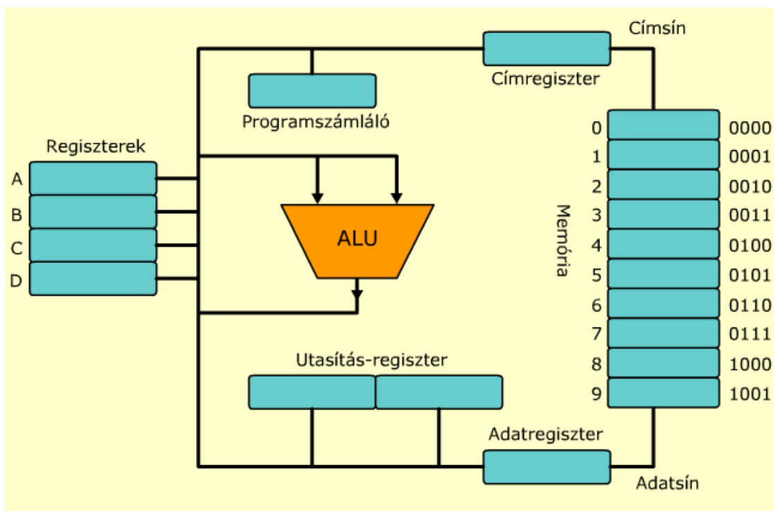
4.6. ábra. Egyszerű processzor-modell.
