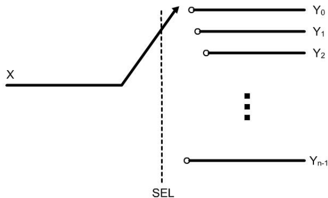
2.29. ábra. Demultiplexer elvi kapcsolása.
