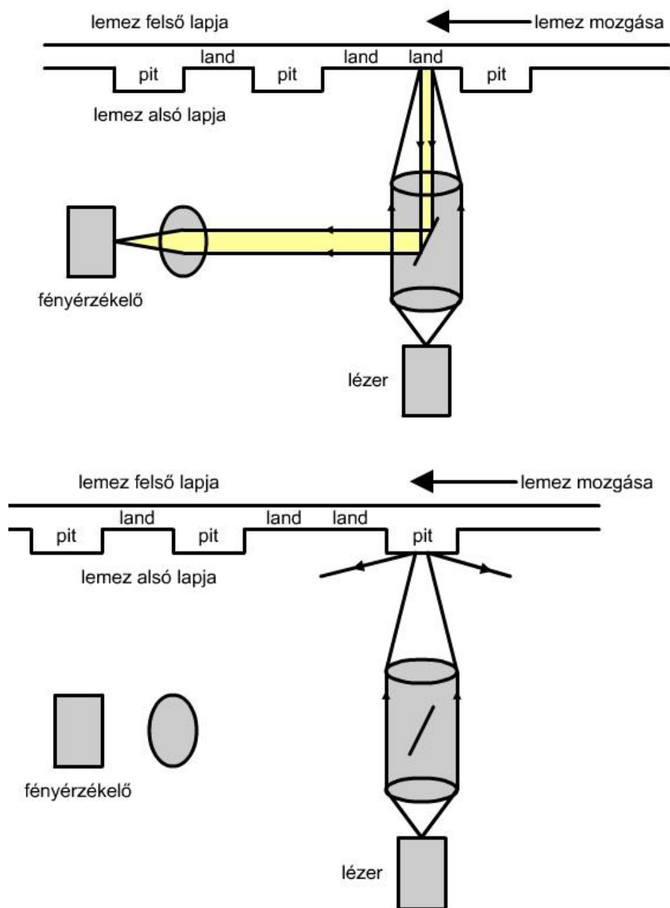
9.3. ábra. A CD-ről való információ olvasása
