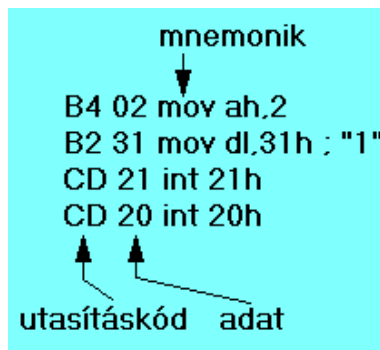
7.7. ábra. Mintaprogram 1 szám nyomtatására.
