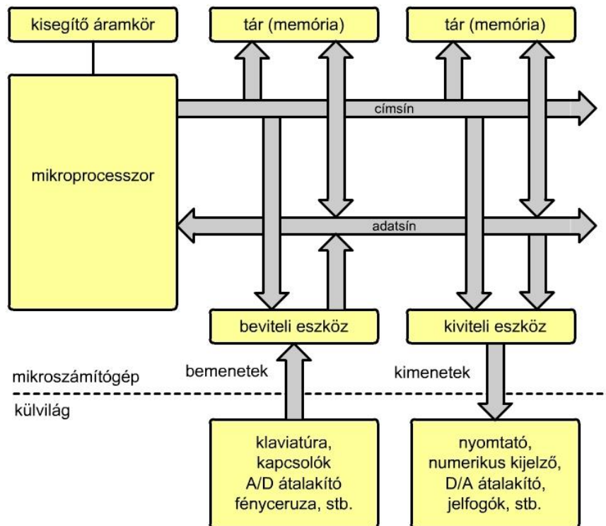
3.19. ábra. A számítógép-rendszer sematikus ábrázolása.
