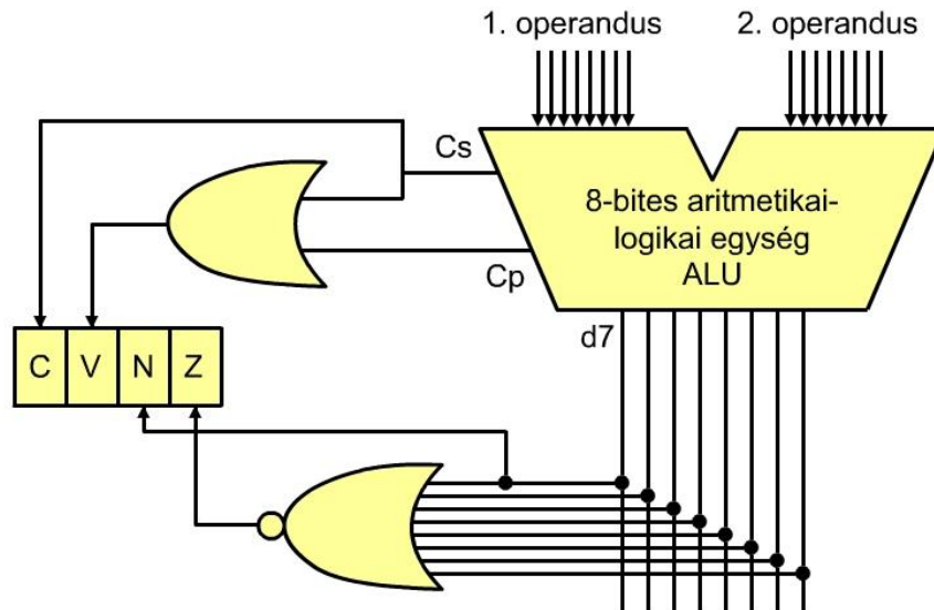
4.31. ábra. A jelzőbitek és az aritmetikai logikai egység kapcsolata.
